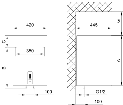
Abb. 1: Senkrechte Montage an die Wand
