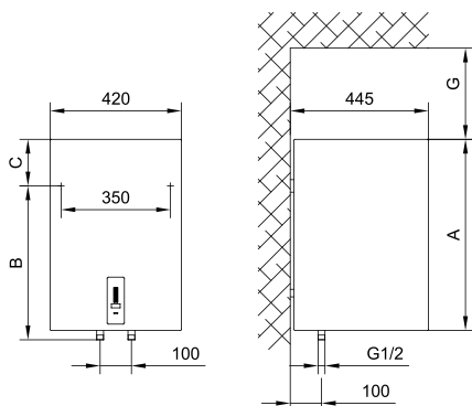
Sl. 1: Uspravno postavljanje na zid
