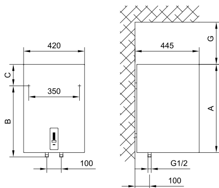
Sl. 1: Pokončna namestitvev na steno
